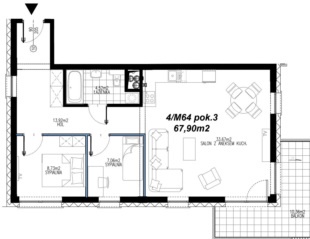
RZUT MIESZKANIA:
